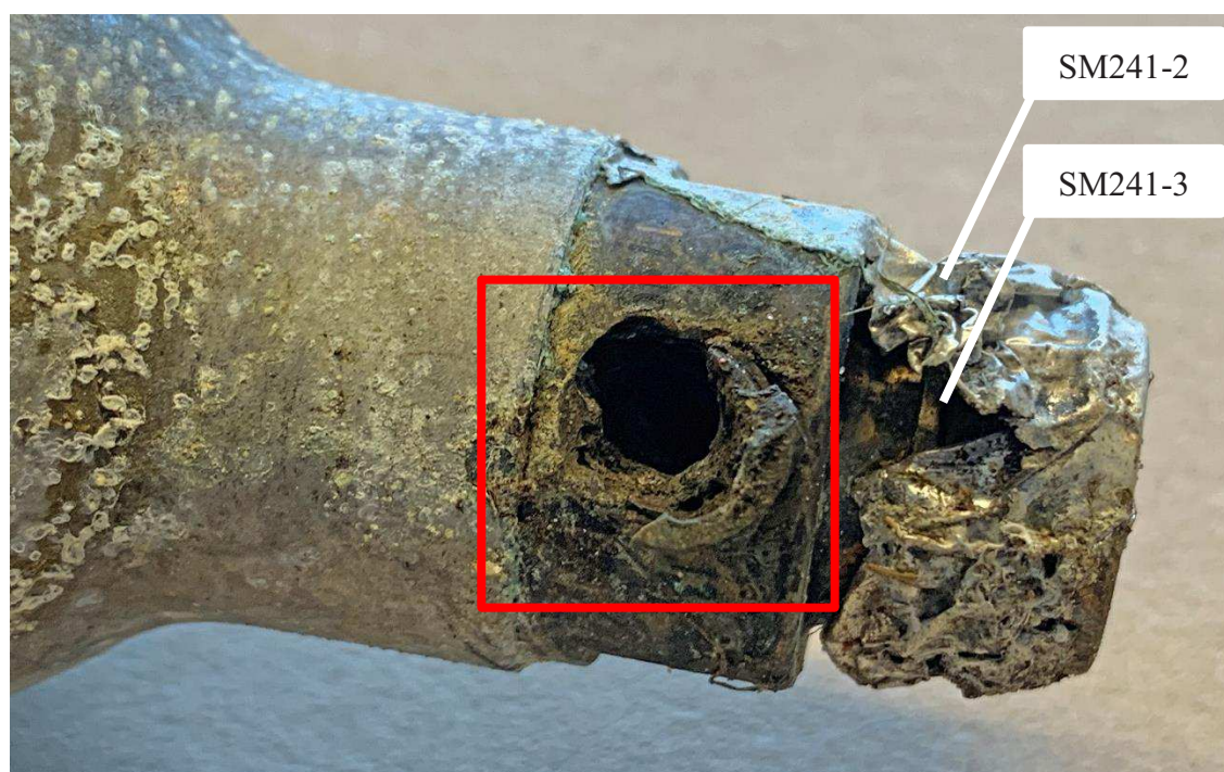
Figur 5. Patronens ventil saknar delar och på ventilen sitter metallfolie. Röd markering visar skruvhålet/gänggången och delen av skruven. SM241-2 och -3 markerade.
