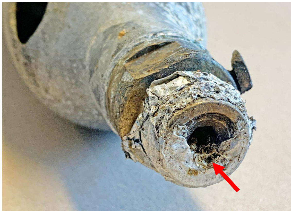
Figur 4. Patronens ventil saknar delar och på ventilen sitter metallfolie. Röd pil markerar var ett stift finns i motsvarande ventil i originalsckick.
