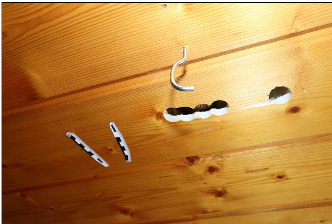
Figur 22. Foto över takkrok efter testet. Infästningen i taket var opåverkad men kroköglan vek upp sig.
