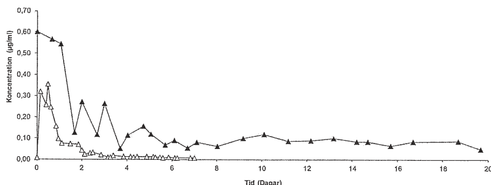
Figur 2. Exempel på utsöndring av THC-syra efter enstaka ( \Delta ) respektive dagligt ( \blacktriangle ) intag av THC.
