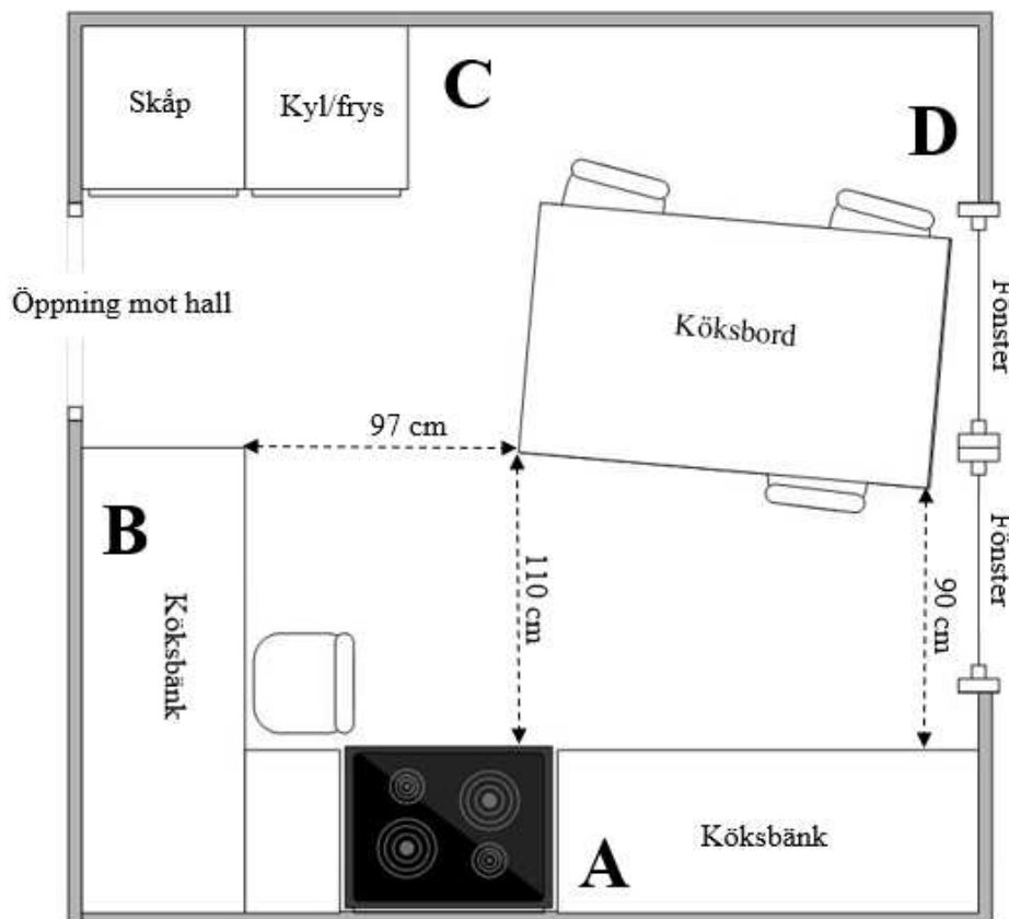
Figur 1. Skiss över köket med sidorna A-D utmärkta. Upprättad 2025-08-01 av Jonas Carlsson.
