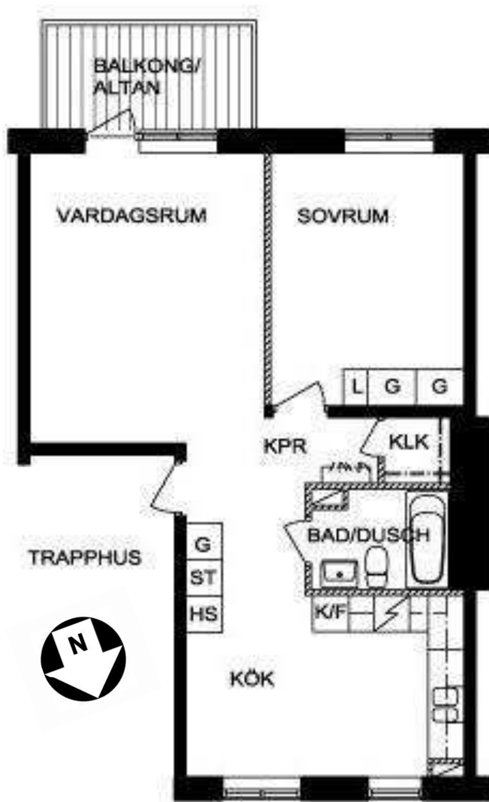
Ritning 1. Ritningen har distribuerats av fastighetsägaren Viktoriahem och redigerats av Jan Enmark.
