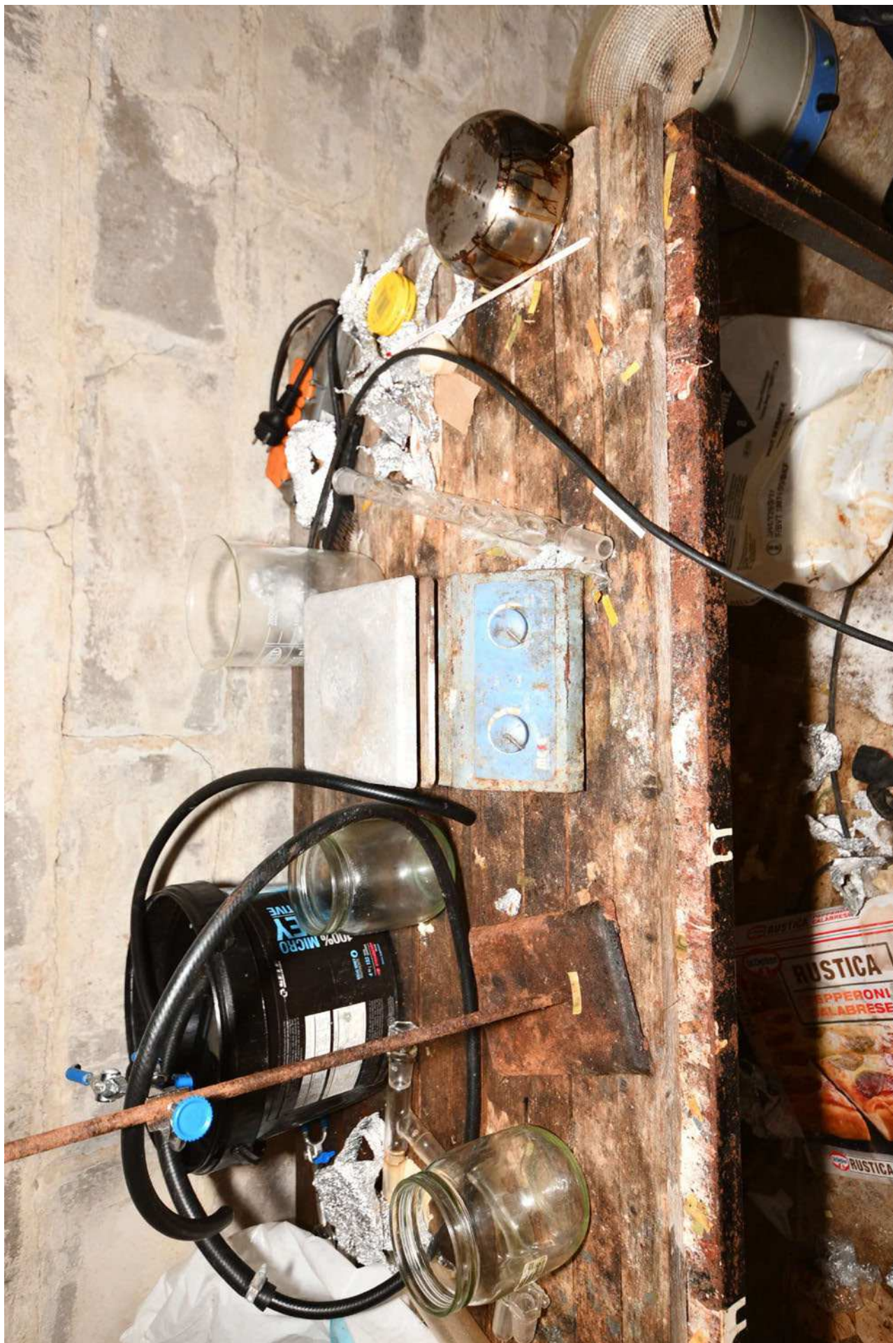
5. Punkten 2 (värmeplatta). Punkten 15 (mätglas 2000 ml som stod på värmeplattan samt delar av punkten 21 (del av syntesutrustning) på labbänk i källaren
