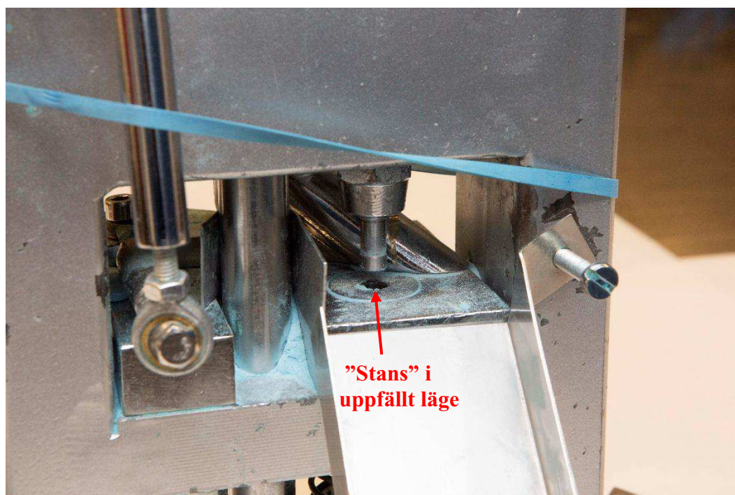
Figur 15. Närbild av maskinens/redskapets "stans" då den är i uppfällt läge.
