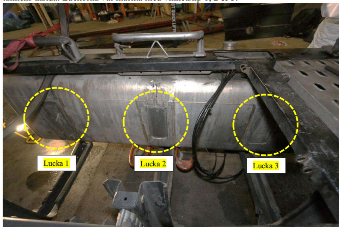
Figur 13. Markeringarna visar de tre dolda luckorna på dieseltankens baksida.
