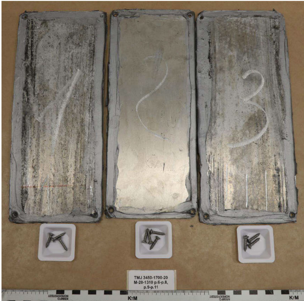
Bild 47. Plåtarna och skruvarna som täckte de konstruerade hålen på baksidan av tanken.
